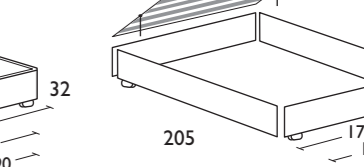
Base smontabile (fissa o sollevabile)
